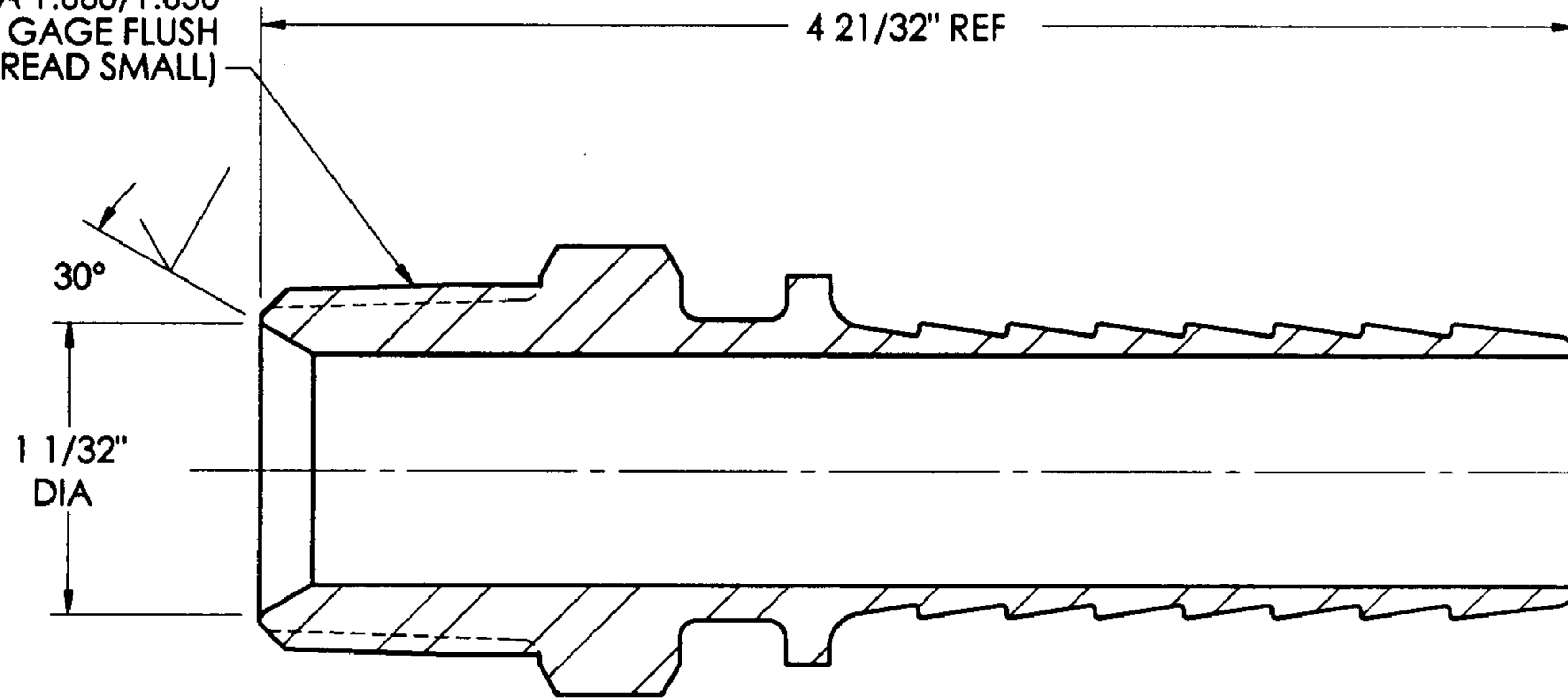
SECTION A-A
